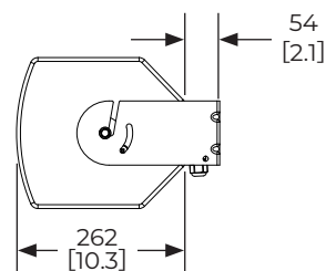
側面 8
