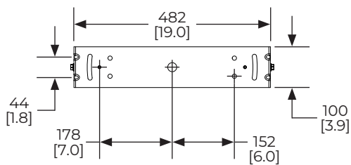
后视图
