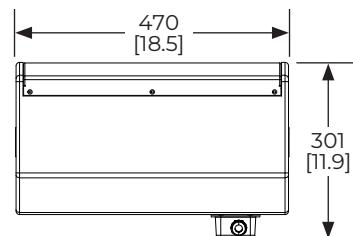
底视图
