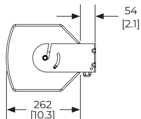
侧视图 8
