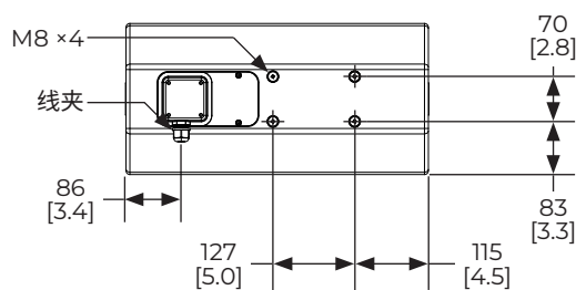
后视图
