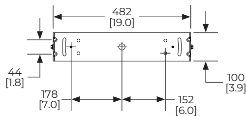
Vista trasera
