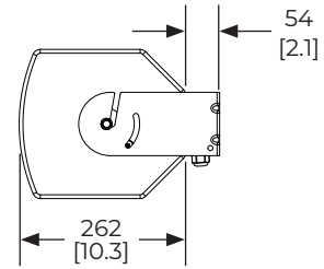
Vista lateral 8
