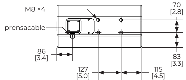
Vista trasera
