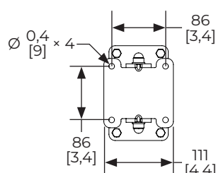
Vue arrière
