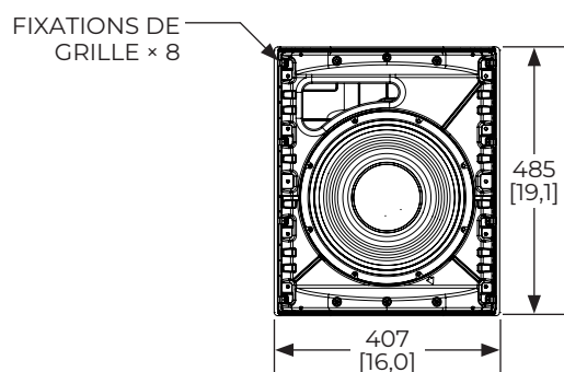
Vue avant
