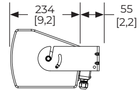
Seitenansicht 8
