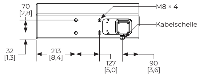
Rückansicht
