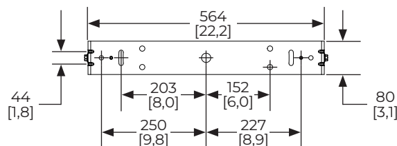
Rückansicht
